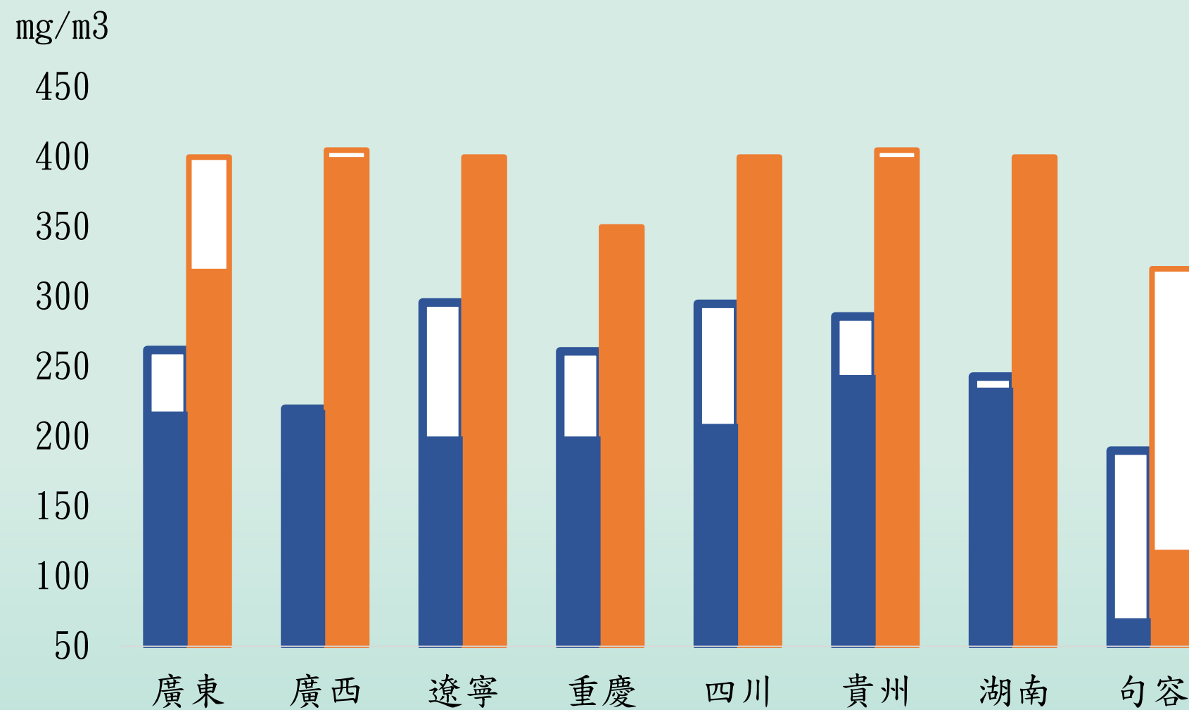
2019Q1 平均 NOx 排放量
